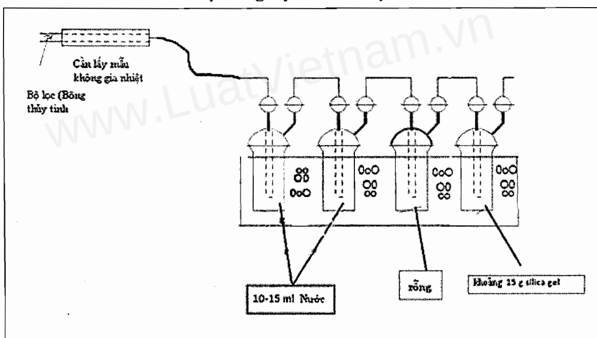
Hình 16: Hệ thống các impinger trong ống khối
