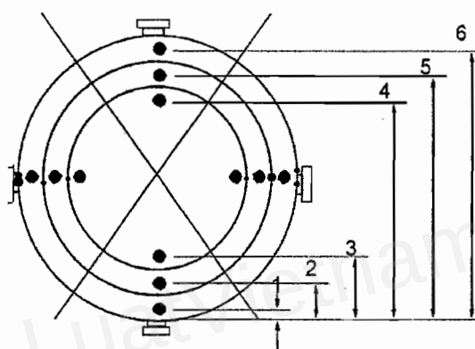
Hình 9: Phân bố 12 điểm hút mẫu đối với ống khối hình tròn
