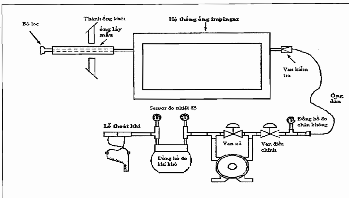
Hình 15: Hệ thống lấy mẫu xác định hàm ẩm
